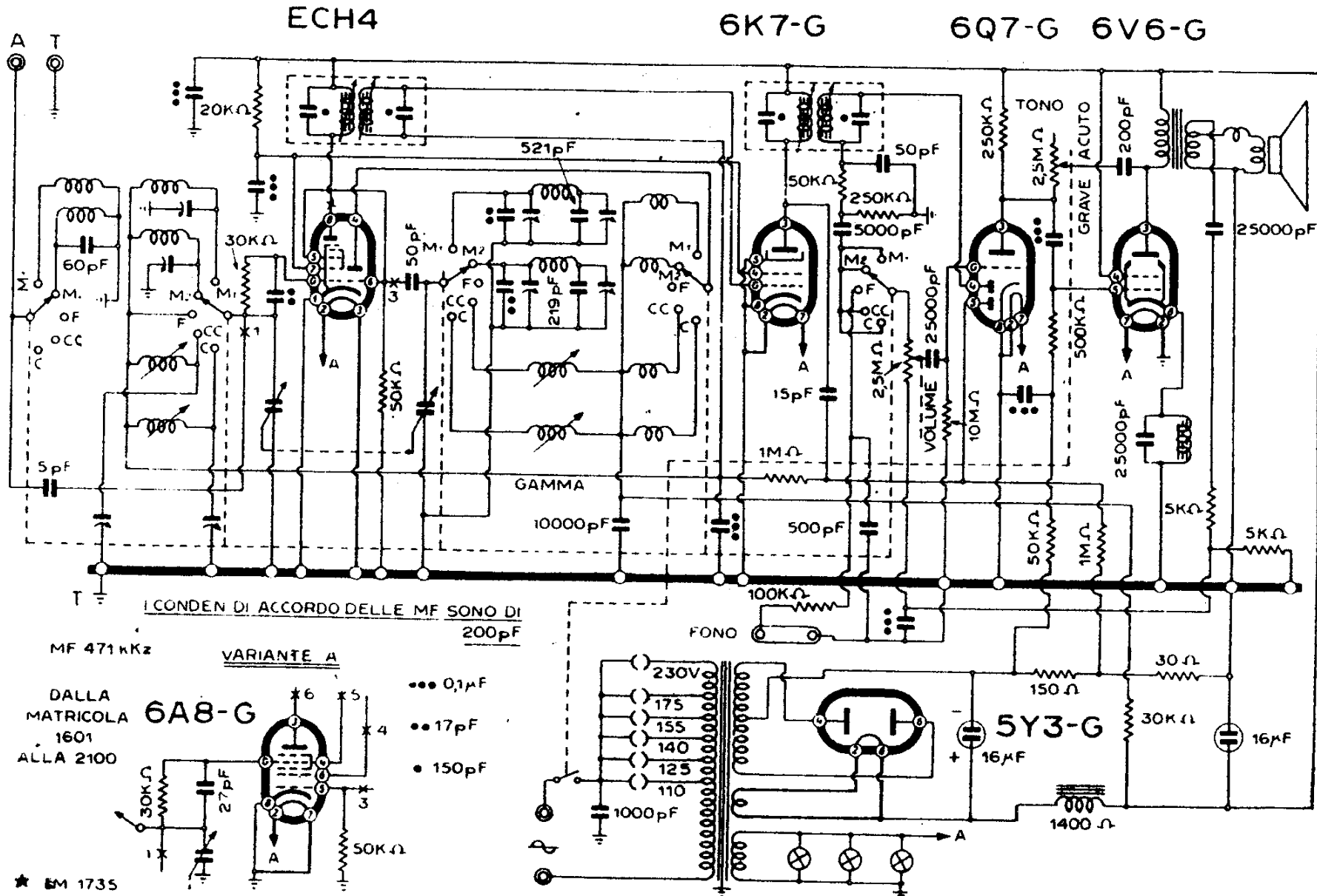
MAGNADYNE - MODD. « SV 64 » « SV 66 »
